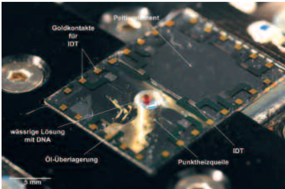
Abb. 1: „Lab-on-a-Chip“: Den Transport der winzigen Probenmengen in ihren ‚virtuellen Reagenzgläsern‘ übernehmen akustische Oberflächenwellen, die von einem Interdigitalen Transducer (IDT) erzeugt werden. Die wässrige Lösung mit dem genetischen Material (rot) wird von einem hauchdünnen Ölfilm vor Verdunstung geschützt. Eine Punktheizquelle und ein Peltierelement sorgen präzise für die Temperaturen, die für die PCR notwendig sind.
